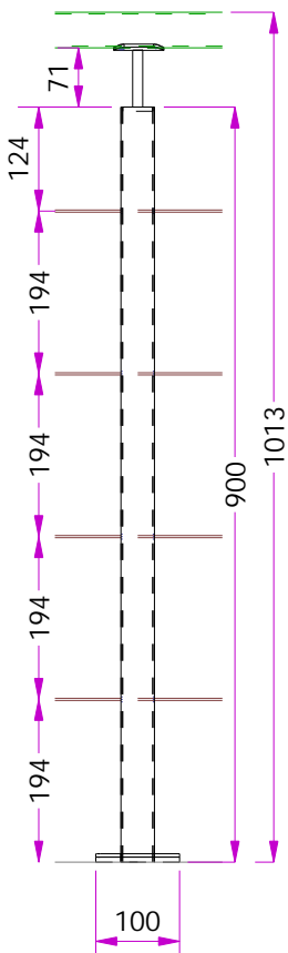
Fragment 1:10
