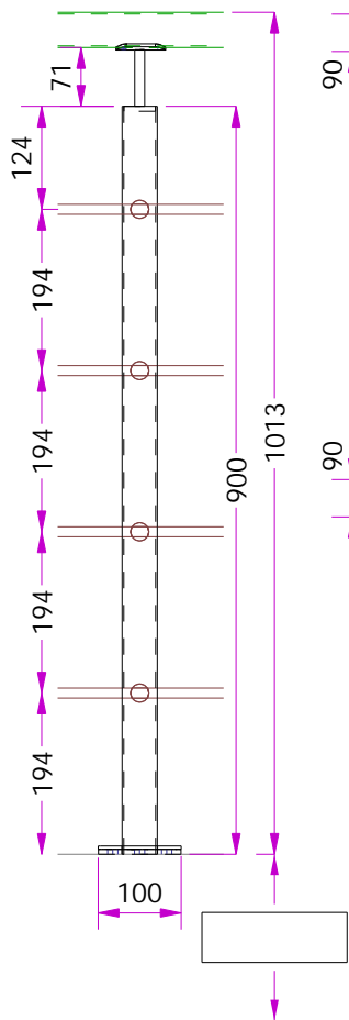
Fragment 1:10
