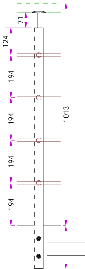
Fragment 1:10
