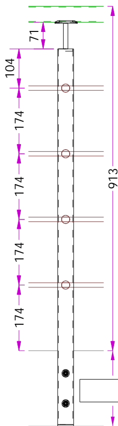
Fragment 1:10
