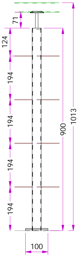
Fragment 1:10
