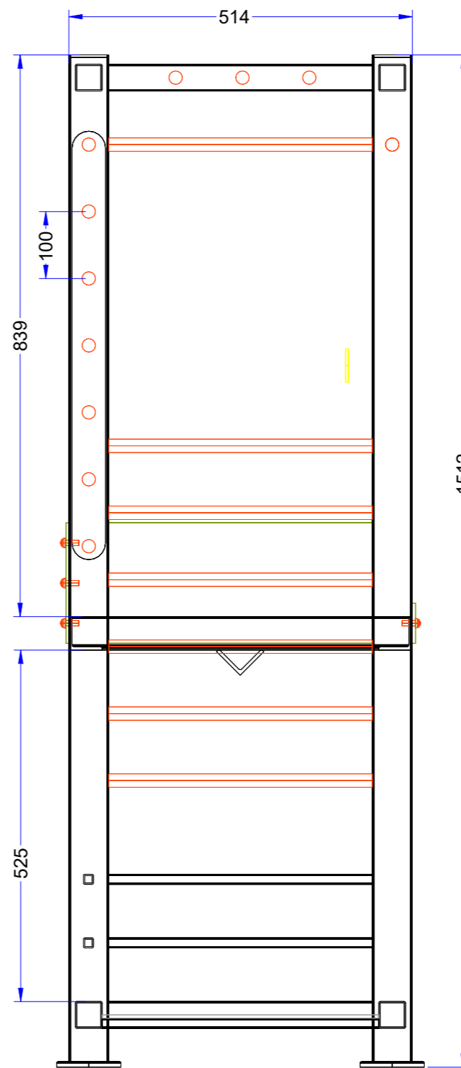
VÄIKE PANN SMG-D20.V.PANN
